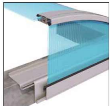
Detalle cabezal cubierta autoportante.
