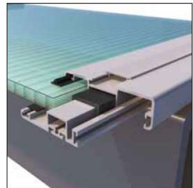
Detalle perfil de aluminio para acabado del punto de partida y de llegada de la cubierta.
