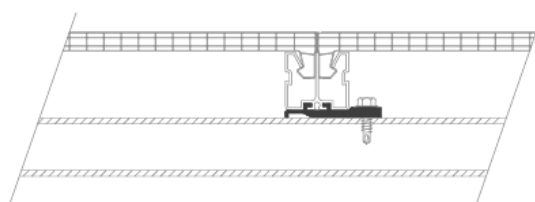
Sección enganche paneles con perfil unión de aluminio
