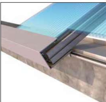
Detalle cubierta autoportante con perfil de unión de aluminio.
